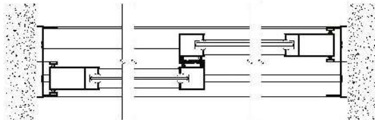
CORTE HORIZONTAL
