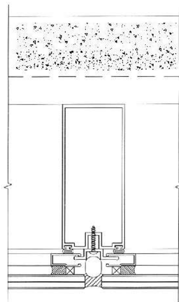
CORTE HORIZONTAL
