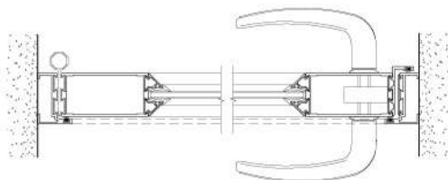
CORTE HORIZONTAL
