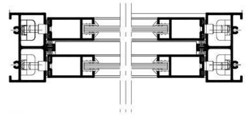
CORTE HORIZONTAL
