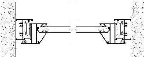
CORTE HORIZONTAL
