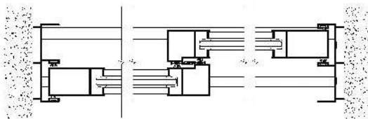
CORTE HORIZONTAL
