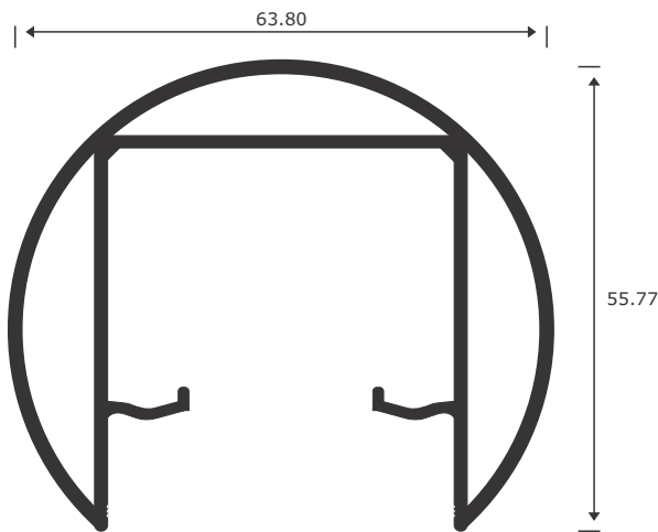
CABEZAL PARA VIDRIO TEMPLADO 8 MM
