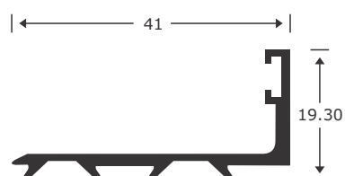
3509 TOPE CON PORTAFELPA
