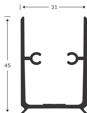
3511 ESCUADRA DE ARMADO
