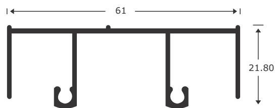
2001 DOBLE RIEL SUPERIOR
