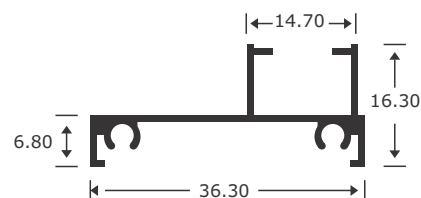
2629 MARCO FIJO
