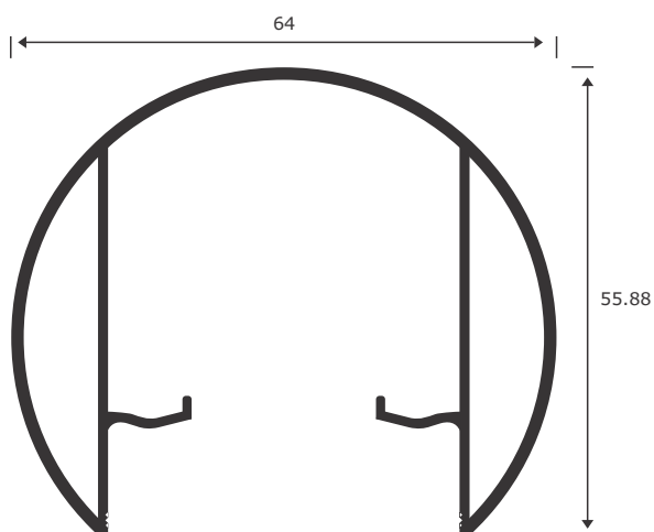
CABEZAL PARA VIDRIO TEMPLADO 6 MM
