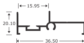
2628 MARCO MOVIL
