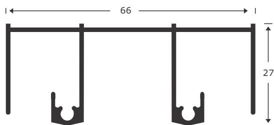
2501 DOBLE RIEL SUPERIOR
