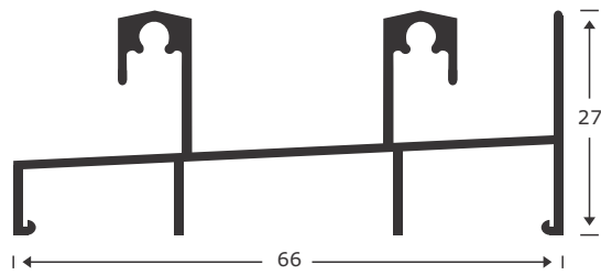
2502 DOBLE RIEL INFERIOR
